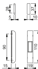
Contacteur solaire radio
